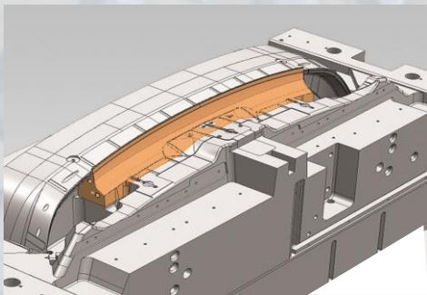
Insert de moule
