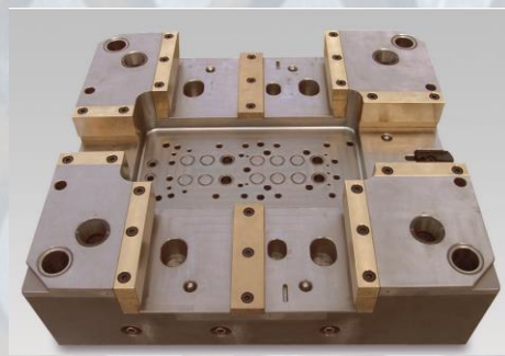
Guidage de coulisse
